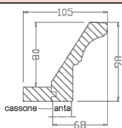
sezione cornice
